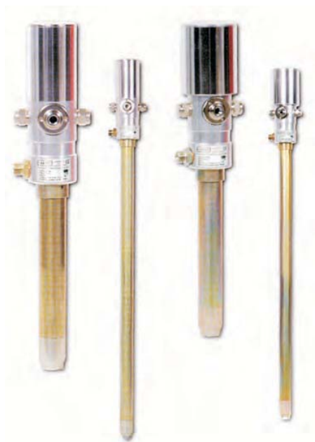
Bomba neumática de aceite, simple efecto
